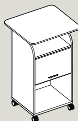
Caddy with a top | Caddy mit Deckplatte | Desserte avec plateau 706 × 630 × 1130 mm
